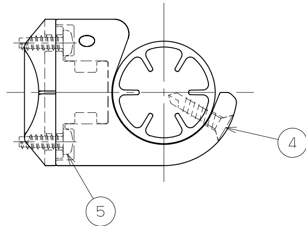
ビーム固定金具納まり図
